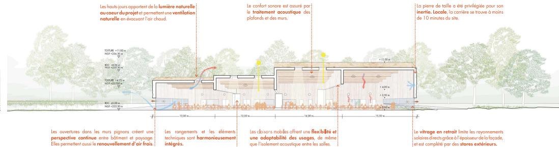
Coupe longitudinale Ech. 1/200 Lorsque les cloisons modulables sont repliées, un vaste espace se développe pour accueillir les événements culturels et viticoles de la ville. Cette configuration permet l'installation de grandes tables. Le positionnement stratégique des offices et des vestiaires optimise l'usage de l'espace, offrant à la fois praticité et efficacité.
