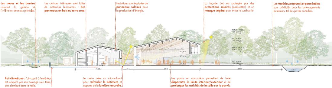
Coupe transversale Ech. 1/200 Le volume de la salle accueille des usages et événements multiples. Ses portes en accordéon s'ouvrent sur le parvis et le faux-plafond permet cette flexibilité de scénarios tandis que le positionnement de la zone artiste simplifie l'accès au fond de scène.
